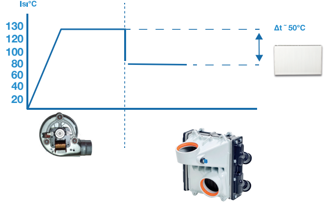
Atık Gaz Isı Grafiği
